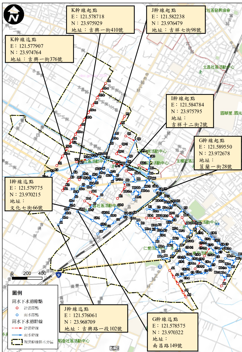
圖 3 宜昌排水區域範圍圖(2)
