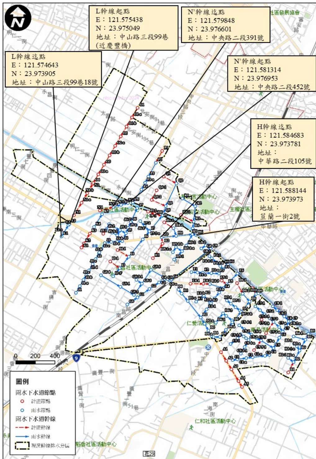
圖 2 宜昌排水區域範圍圖(1)
