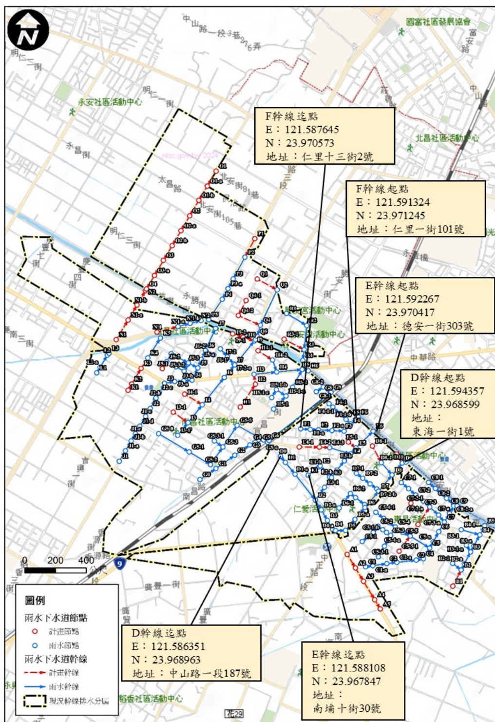
圖 4 仁里各排水區域範圍圖
