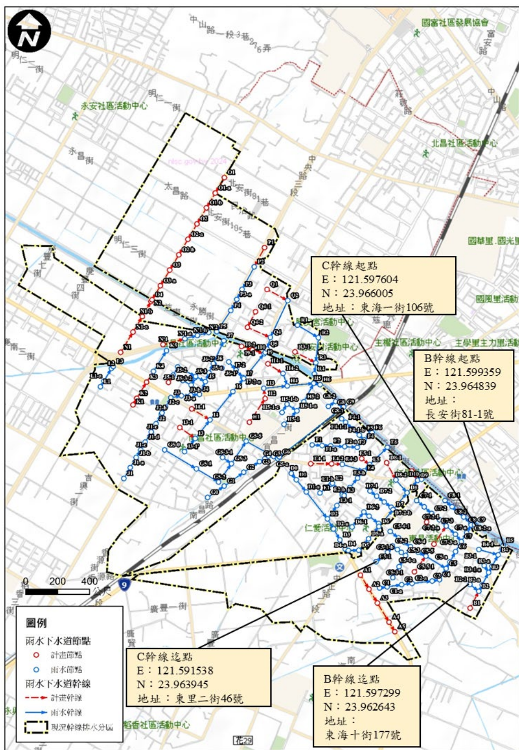
圖 5 仁化排水區域範圍圖
